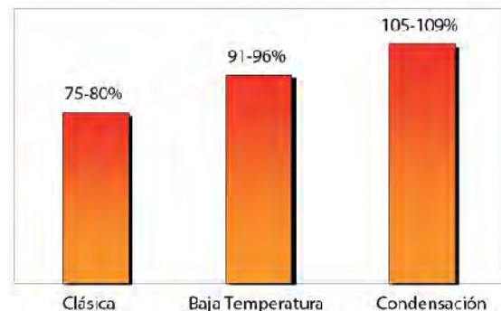
Rendimientos en función de la tecnología de las calderas
