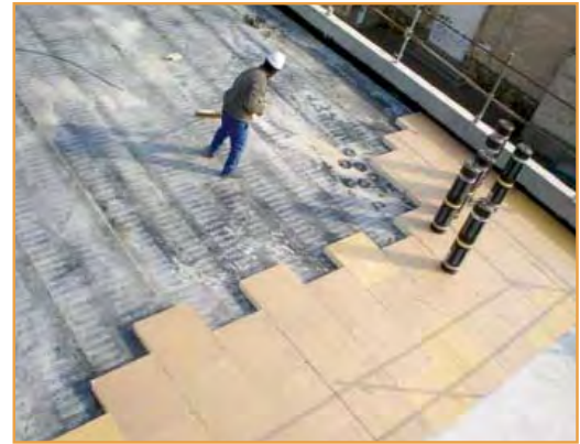
Rehabilitación de cubierta por el exterior
